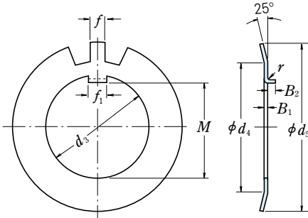
Bent-Tab
